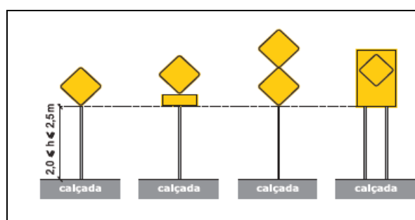
Figura 7.12 – Forma de instalação de placas de advertência
